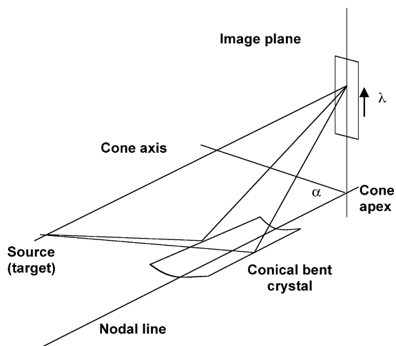
Fig. 1. Spectrometer schema.
