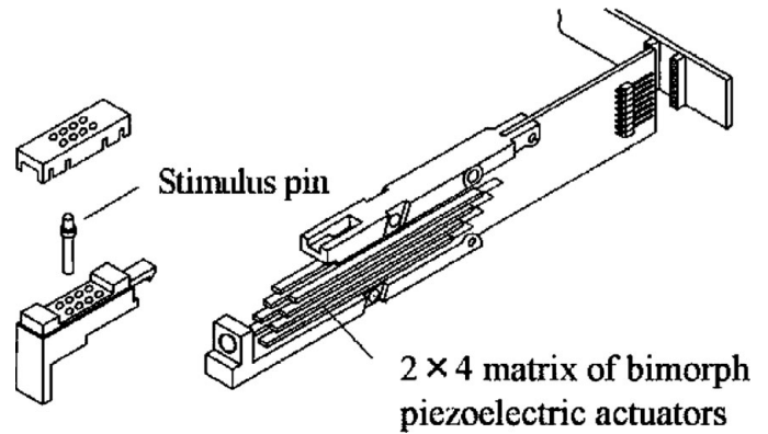
Fig. 1. Braille dot cell (KGS Co., SC-2).
