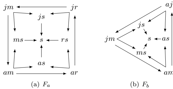
Fig. 2. Argumentation frameworks for SRP.
