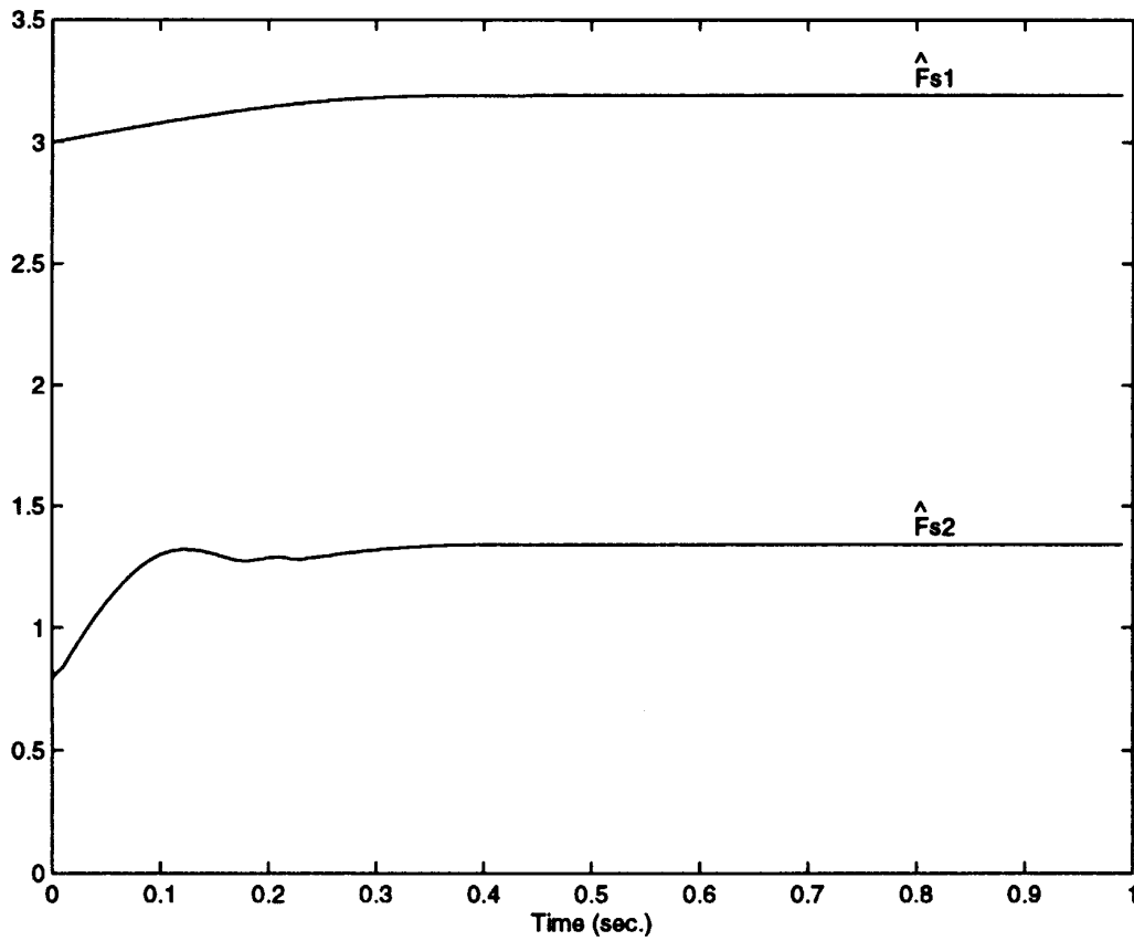
Fig. 5. Parameter estimates.
